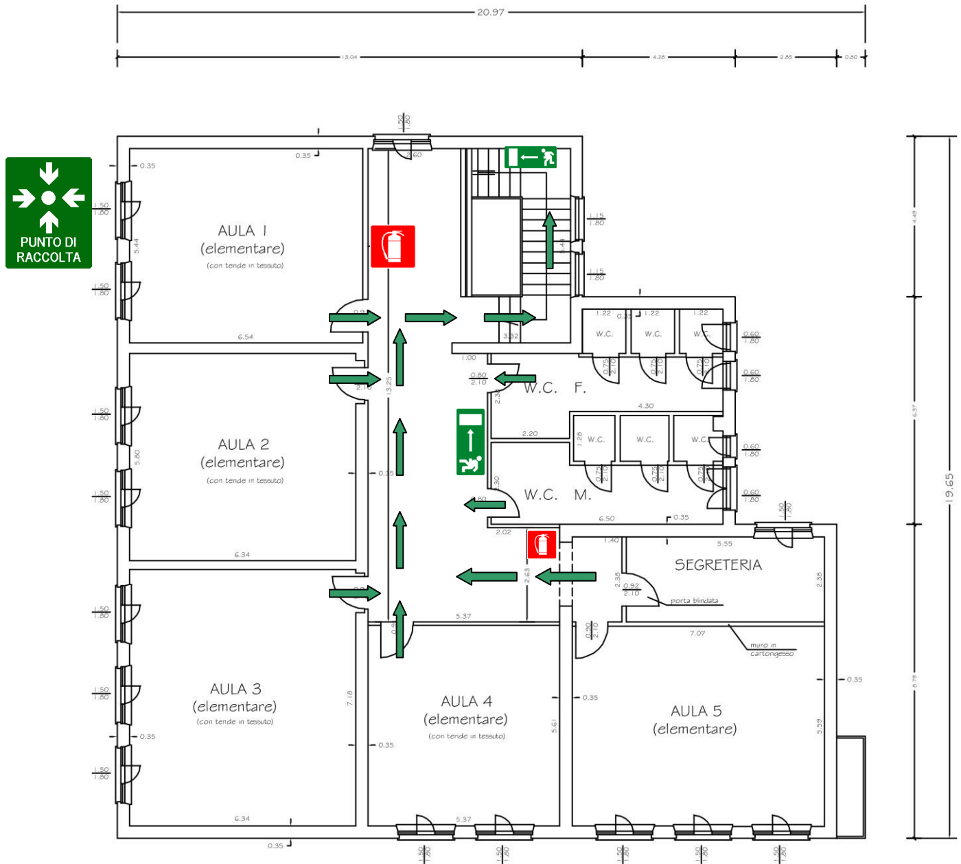
PIANTA PIANO PRIMO - esistente (h interna = 3.25 mt.)
